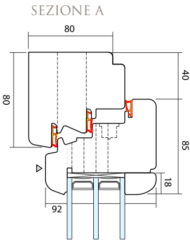
SEZIONE A
