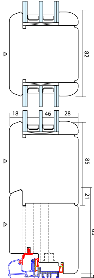
SEZIONE B ALLUMINIO BASSO
