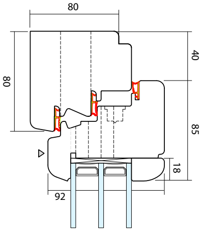
SEZIONE A
