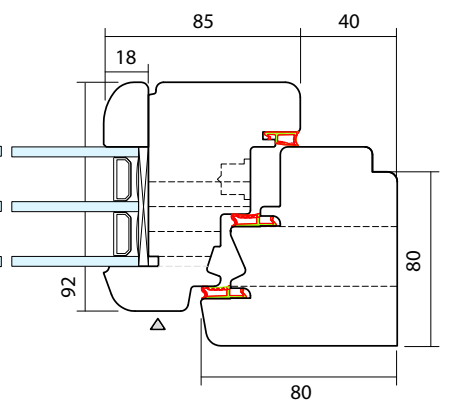
SEZIONE E
