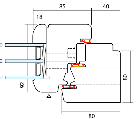
SEZIONE E
