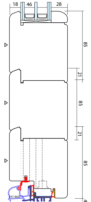
SEZIONE B ALLUMINIO BASSO
