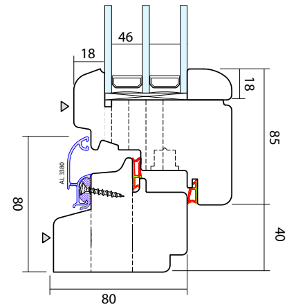
SEZIONE B CON GOCCILOTOIO IN ALLUMINIO
