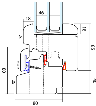
SEZIONE B CON GOCCILOTOIO IN LEGNO
