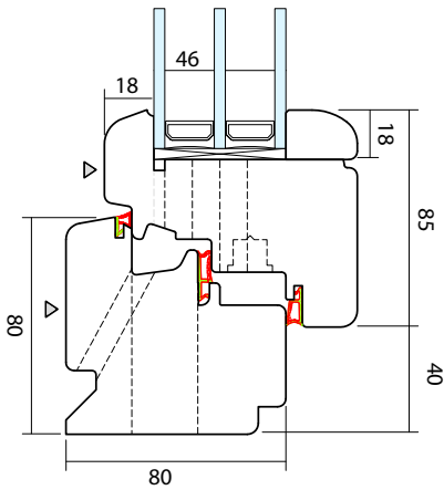
SEZIONE B TUTTO LEGNO
