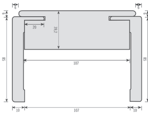
Particolare TELAIO con RINGROSSO "A"
