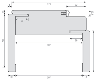
Particolare PASSATA e con ingresso "A"
